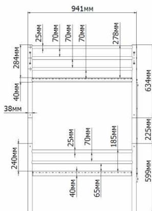
Вид сбоку (1 : 10)
