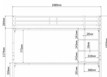
Вид спереди (1 : 10)
