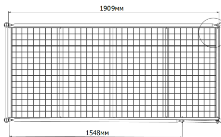
Вид сбоку (1 : 10)
