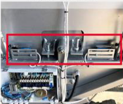
Кінцеві вимикачі
